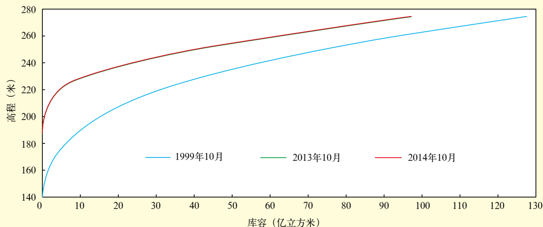
图2-6 小浪底水库库容曲线
