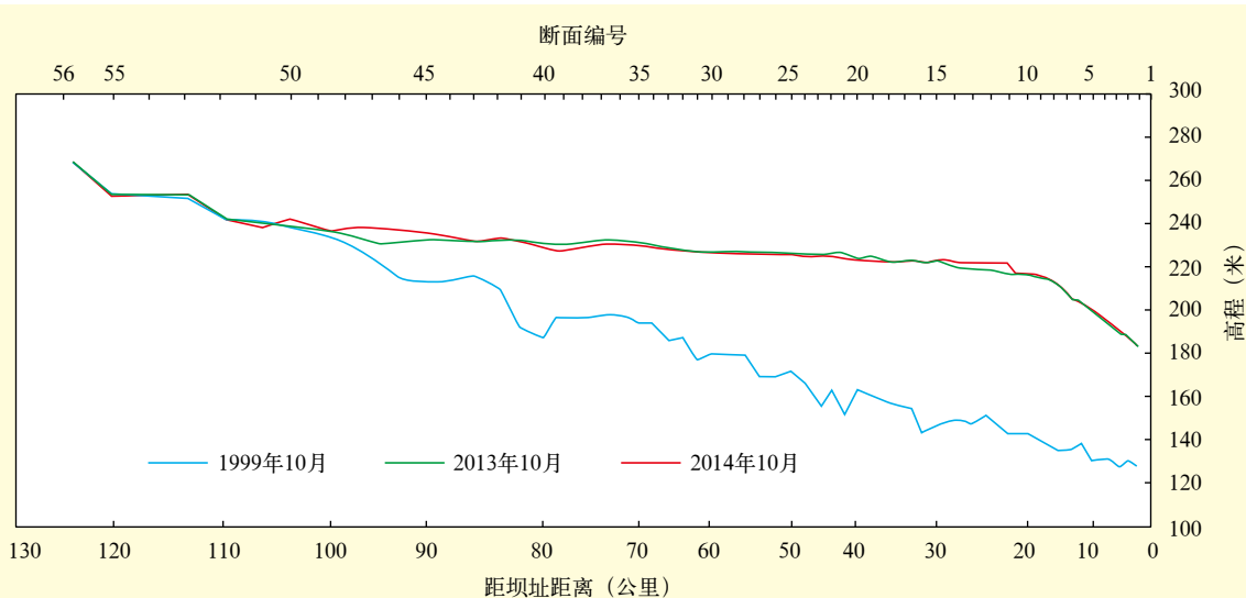
图2-7 小浪底水库深泓纵剖面变化
