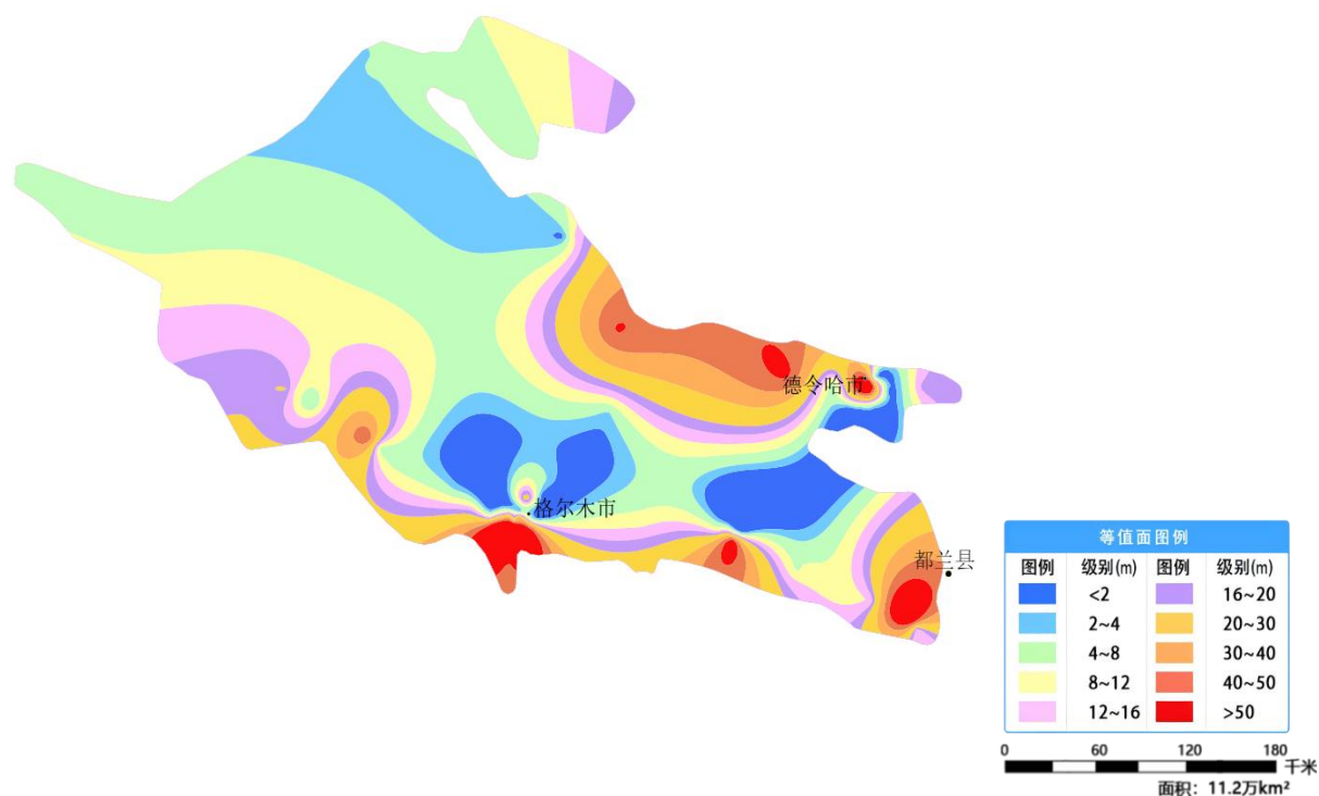
图 26 青海柴达木盆地 12 月份地下水埋深等值面图
