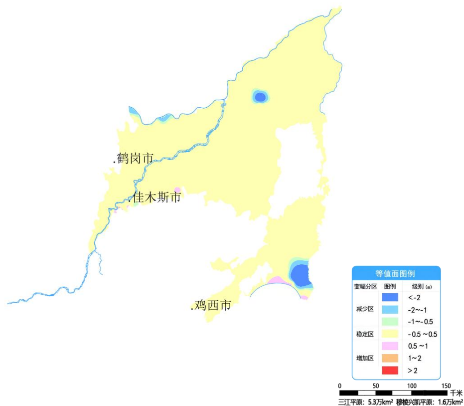
图 2 三江平原和穆棱兴凯平原 12 月份与上月相比地下水埋深变幅图
