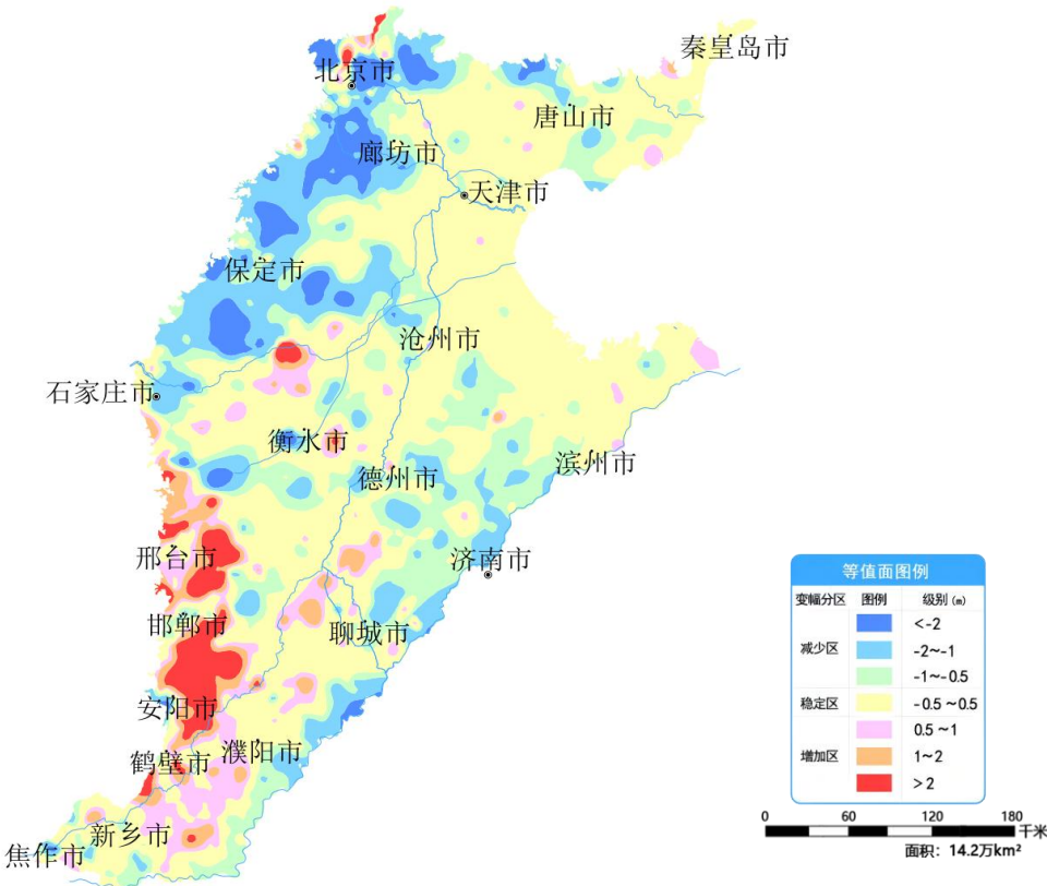
图 12 海河平原 12 月份与去年同期相比地下水埋深变幅图
