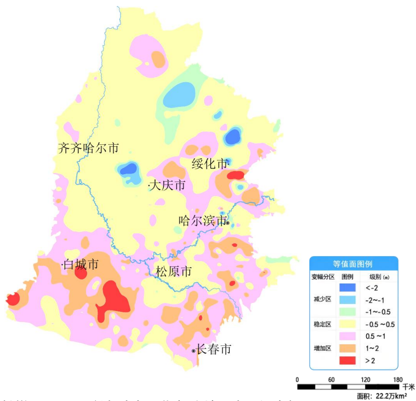
图 6 松嫩平原 12 月份与去年同期相比地下水埋深变幅图
