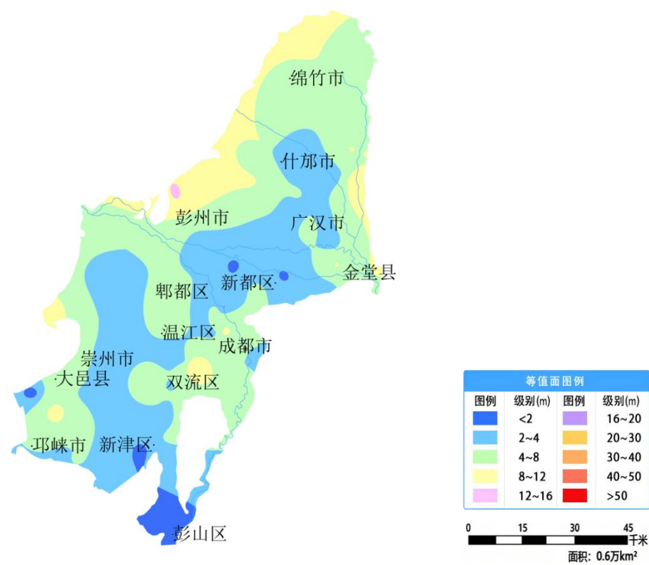
图 32 成都平原 12 月份地下水埋深等值面图
