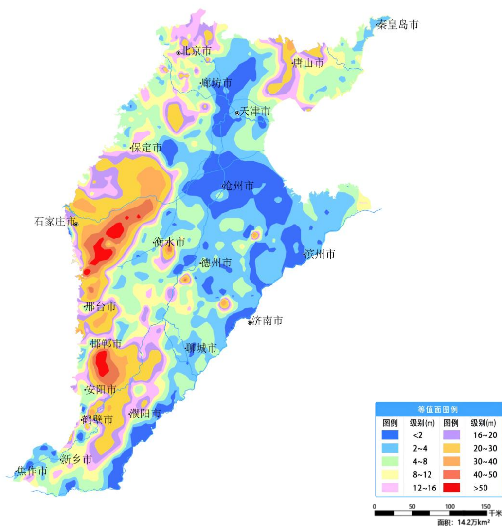
图 10 海河平原 12 月份地下水埋深等值面图
