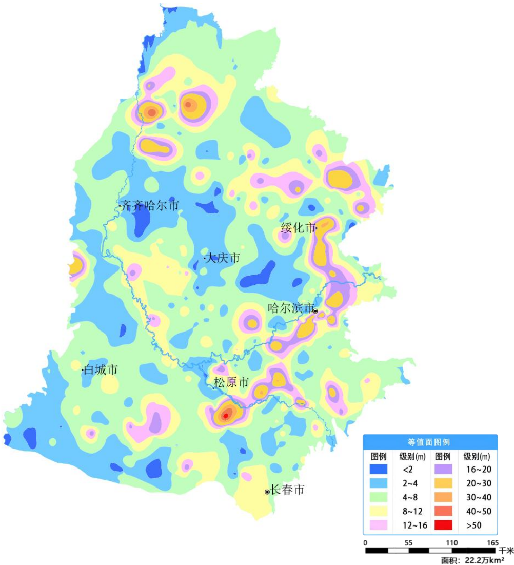
图 4 松嫩平原 12 月份地下水埋深等值面图
