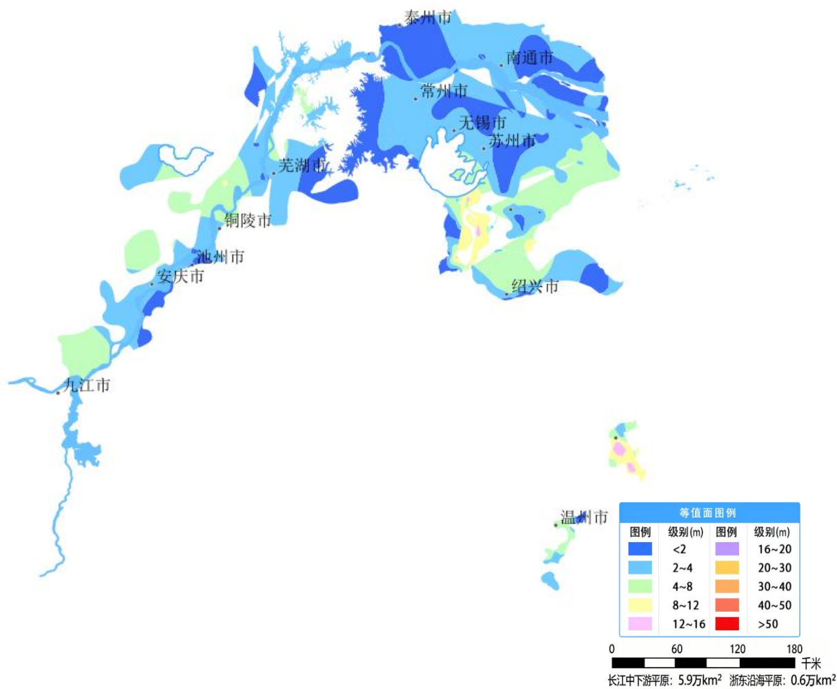
图 30 长江三角洲平原和浙东沿海平原 12 月份地下水埋深等值面图
