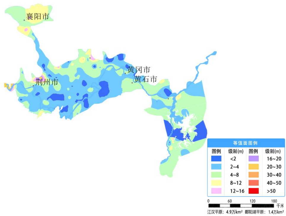
图 29 江汉平原和鄱阳湖平原 12 月份地下水埋深等值面图
