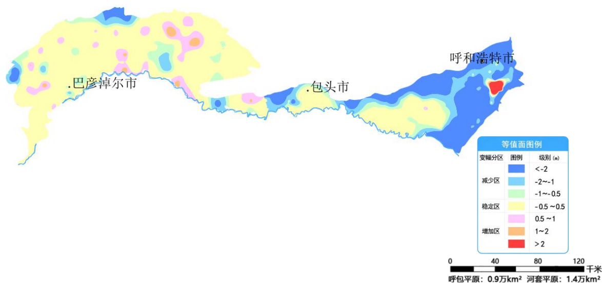
图 18 内蒙古呼包平原及河套平原 12 月份与去年同期相比地下水埋深变幅图
