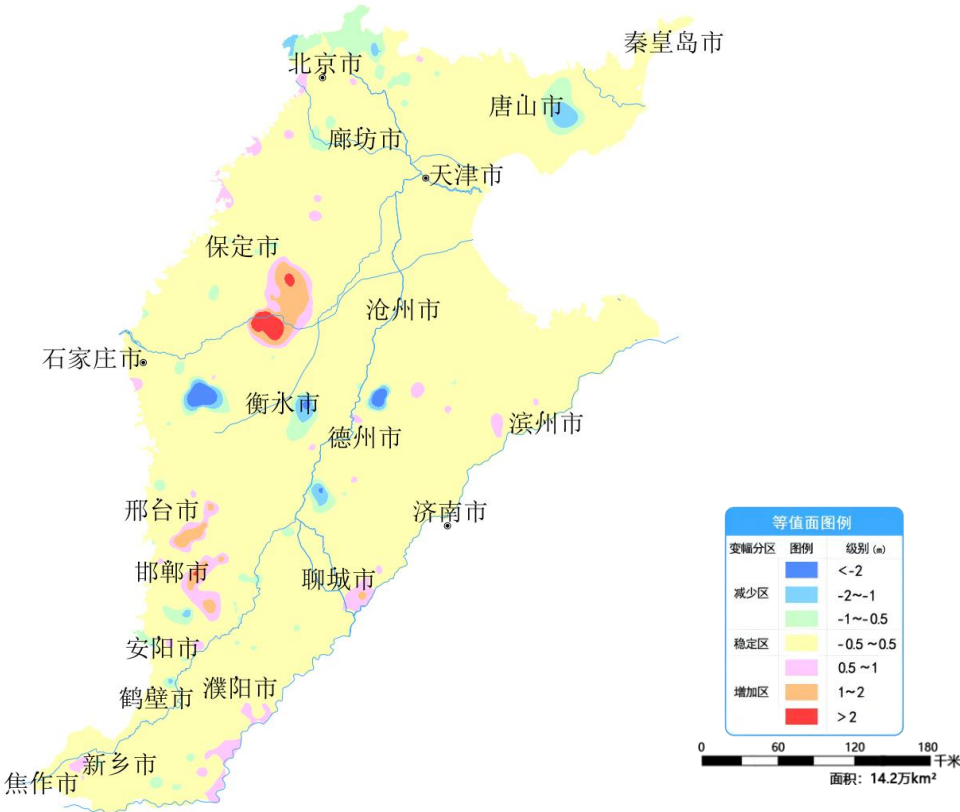
图 11 海河平原 12 月份与上月相比地下水埋深变幅图
