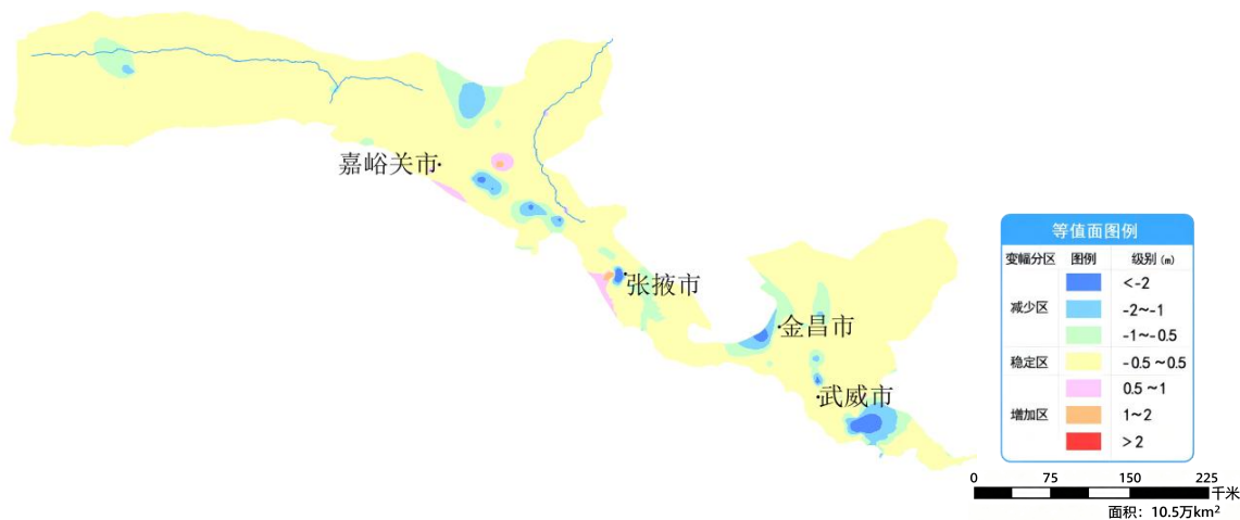
图 23 甘肃河西走廊平原 12 月份与上月相比地下水埋深变幅图
