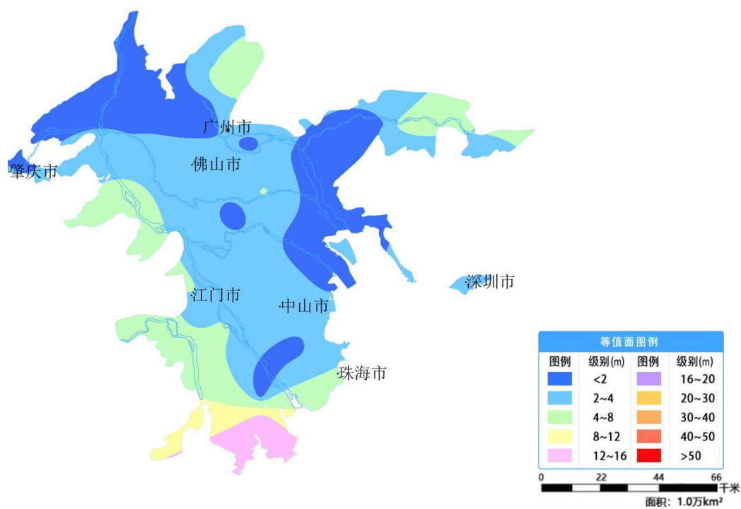
图 33 广东珠江三角洲平原 12 月份地下水埋深等值面图
