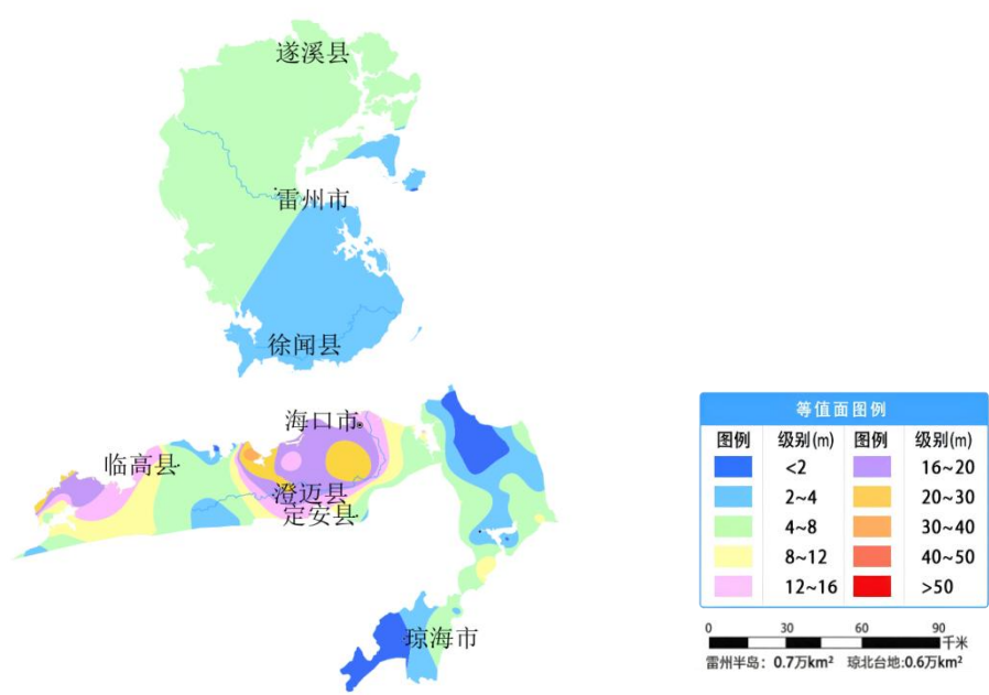
图 34 雷州半岛平原和琼北台地平原 12 月份地下水埋深等值面图
