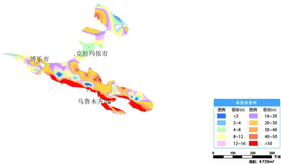
图 28 新疆准噶尔盆地监控区 12 月份地下水埋深等值面图
