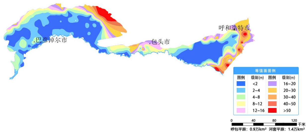
图 16 内蒙古呼包平原及河套平原 12 月份地下水埋深等值面图
