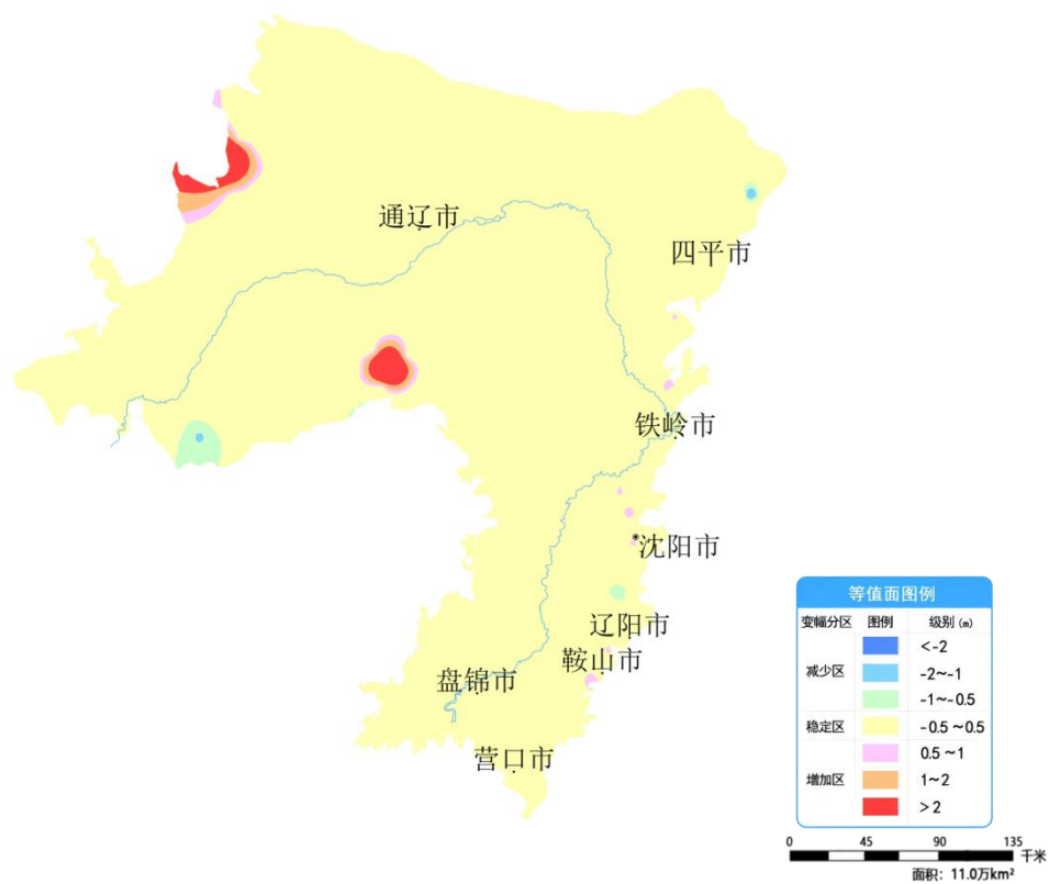
图 8 辽河平原 12 月份与上月相比地下水埋深变幅图
