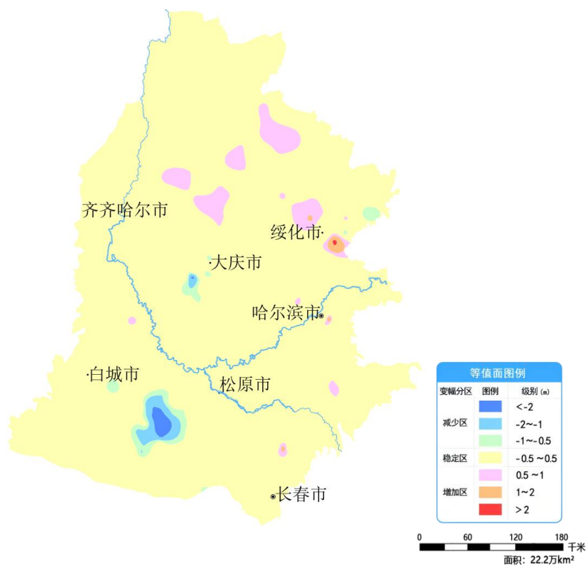
图 5 松嫩平原 12 月份与上月相比地下水埋深变幅图
