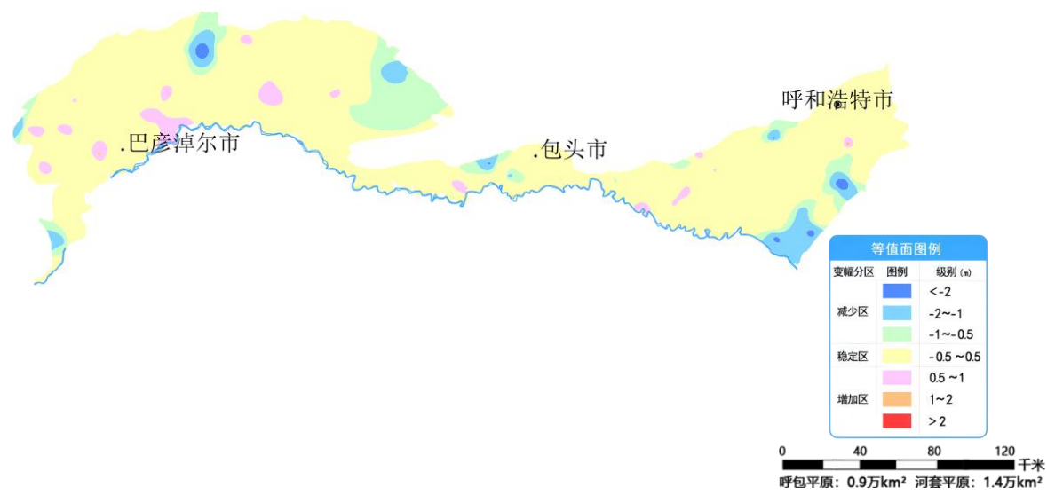
图 17 内蒙古呼包平原及河套平原 12 月份与上月相比地下水埋深变幅图
