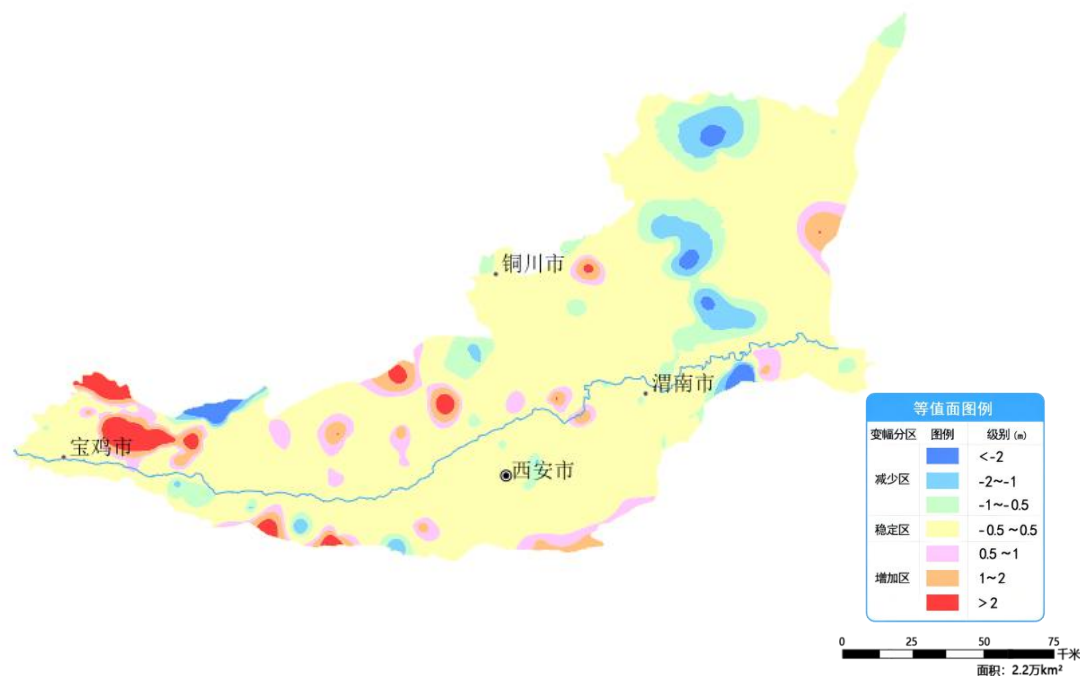
图 20 陕西关中平原 12 月份与上月相比地下水埋深变幅图
