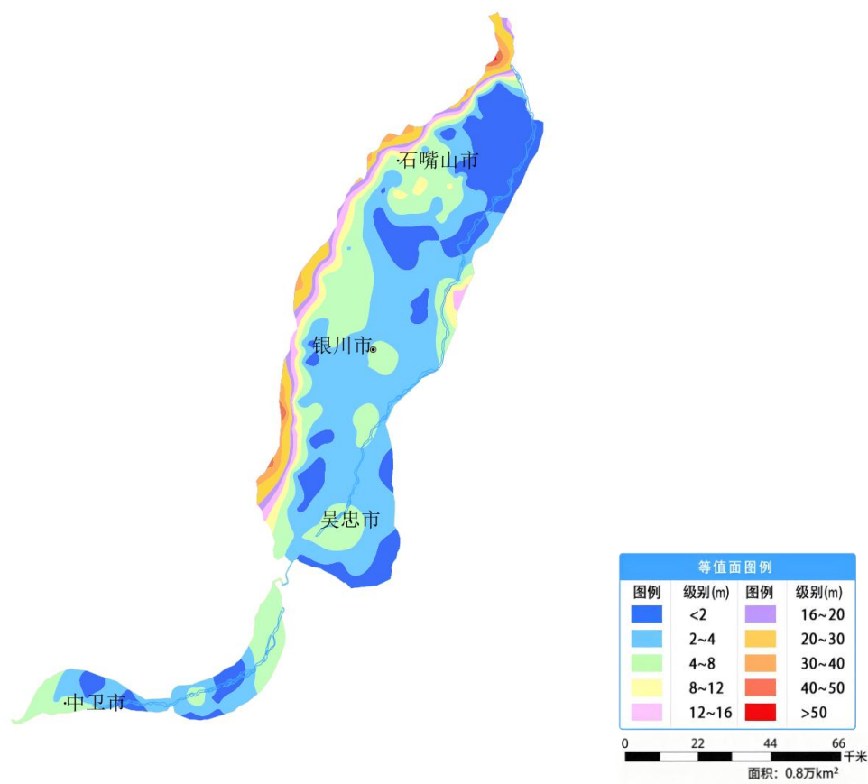
图 25 宁夏银川卫宁平原 12 月份地下水埋深等值面图
