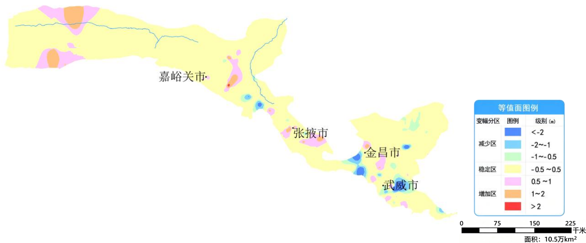
图 24 甘肃河西走廊平原 12 月份与去年同期相比地下水埋深变幅图
