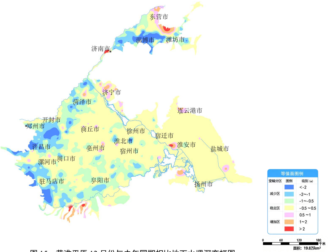
图 15 黄淮平原 12 月份与去年同期相比地下水埋深变幅图
