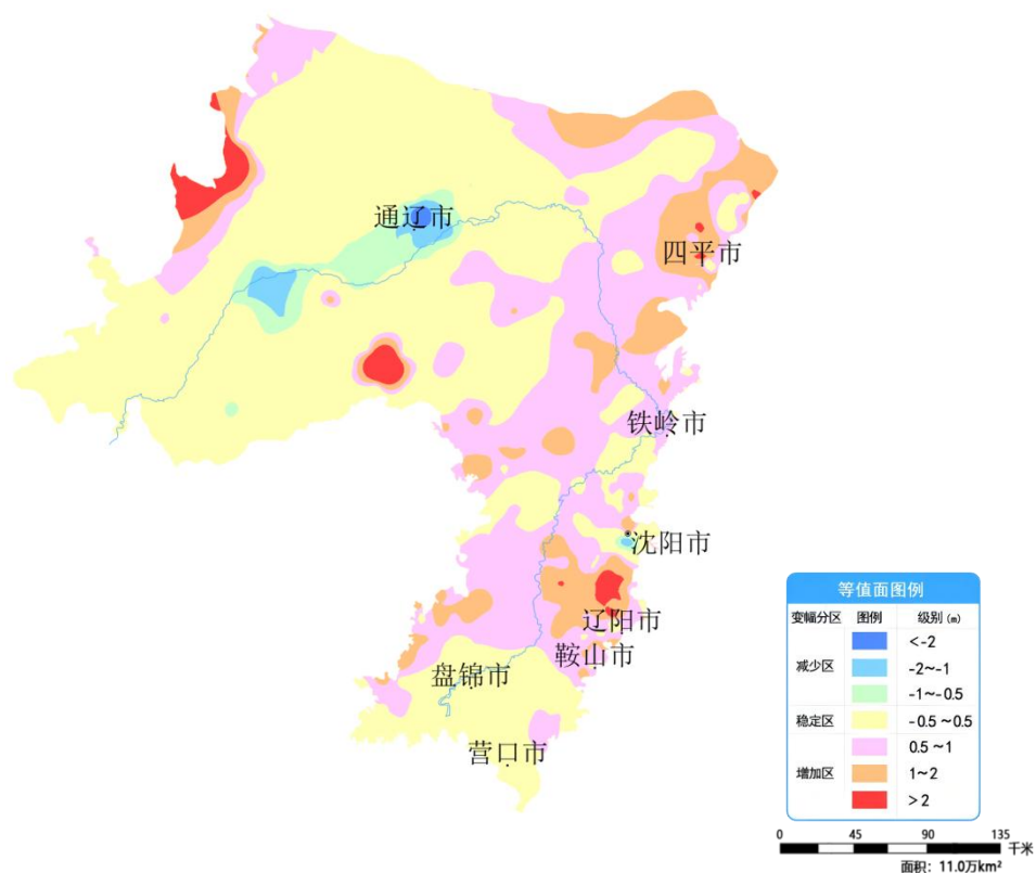
图 9 辽河平原 12 月份与去年同期相比地下水埋深变幅图
