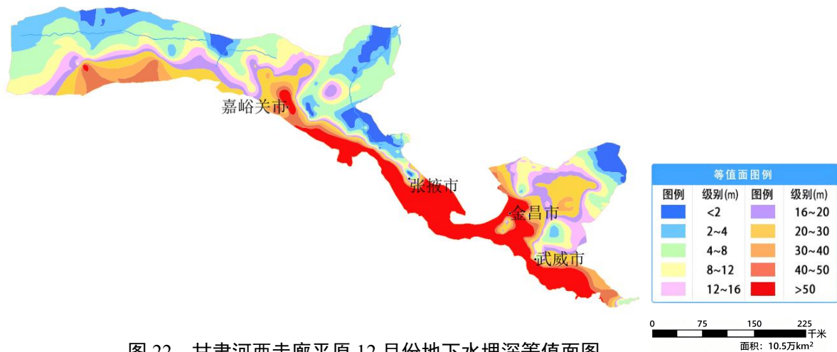
图 22 甘肃河西走廊平原 12 月份地下水埋深等值面图
