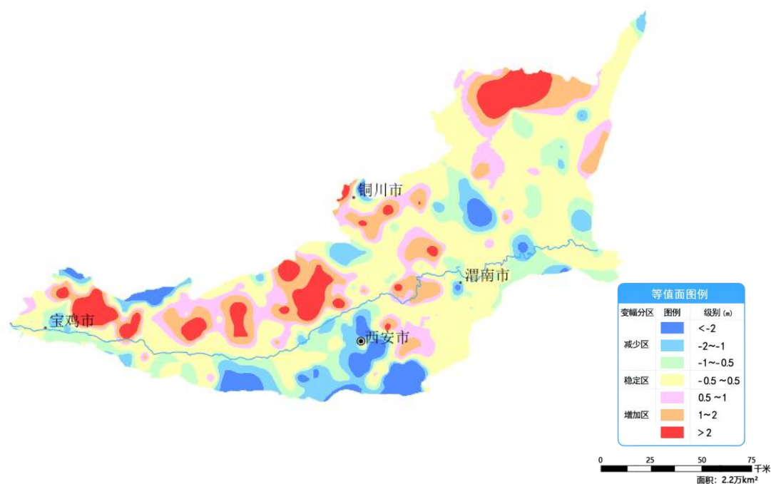
图 21 陕西关中平原 12 月份与去年同期相比地下水埋深变幅图
