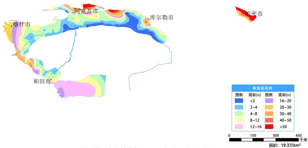
图 27 新疆塔里木盆地监控区 12 月份地下水埋深等值面图
