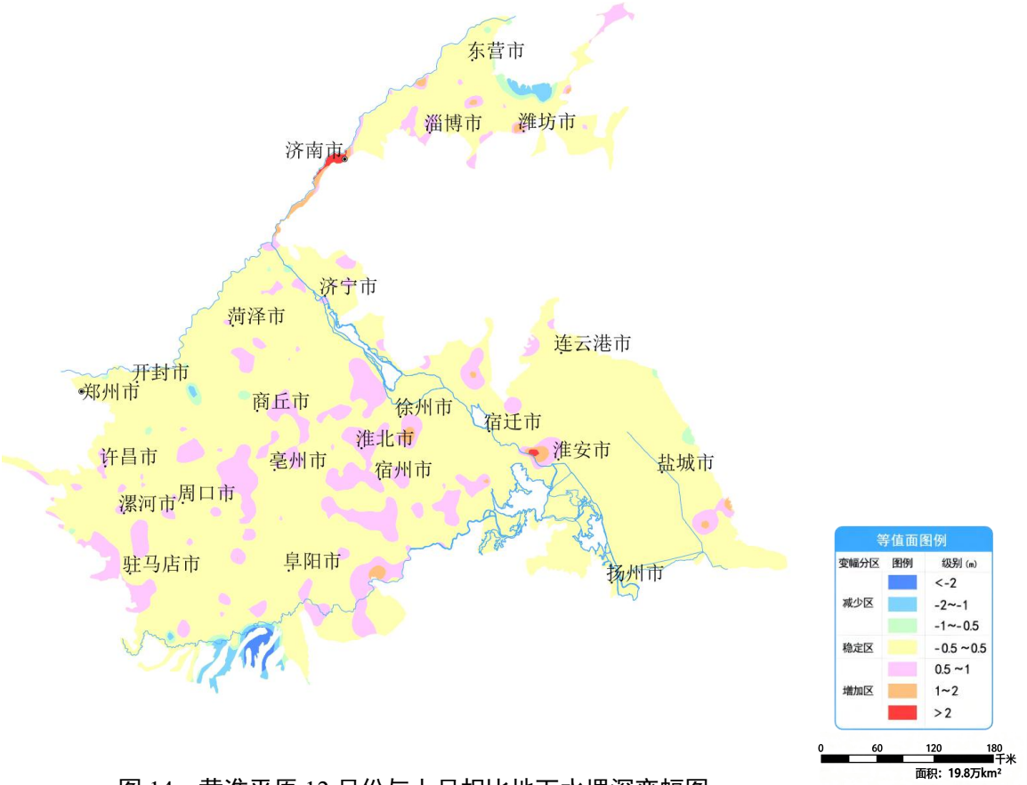
图 14 黄淮平原 12 月份与上月相比地下水埋深变幅图
