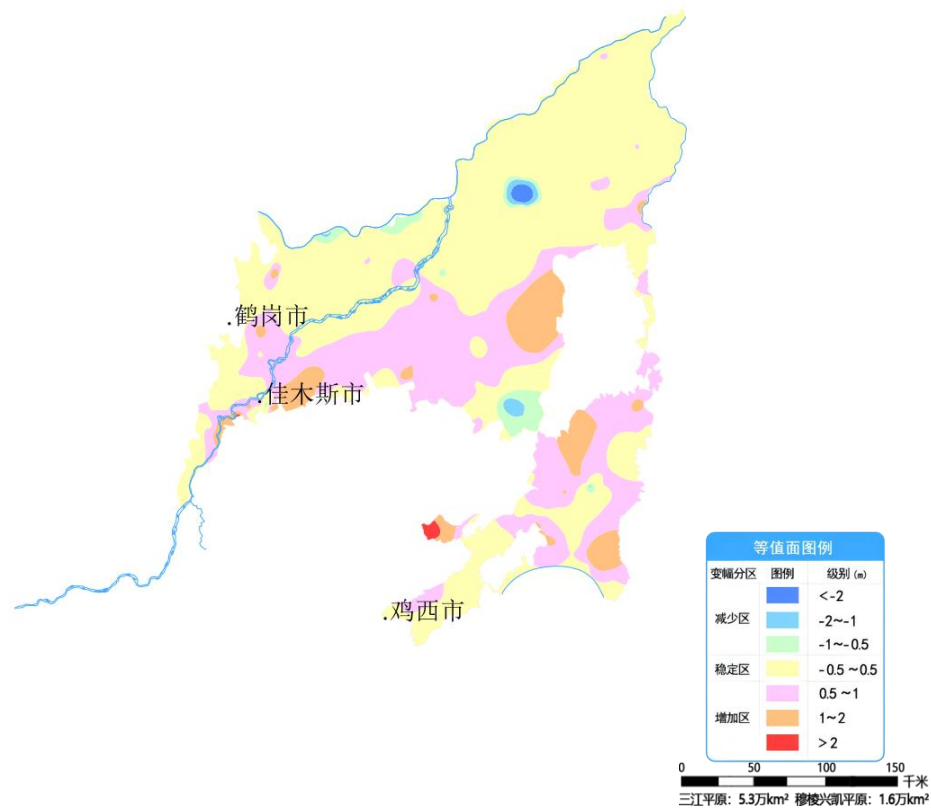
图 3 三江平原和穆棱兴凯平原 12 月份与去年同期相比地下水埋深变幅图
