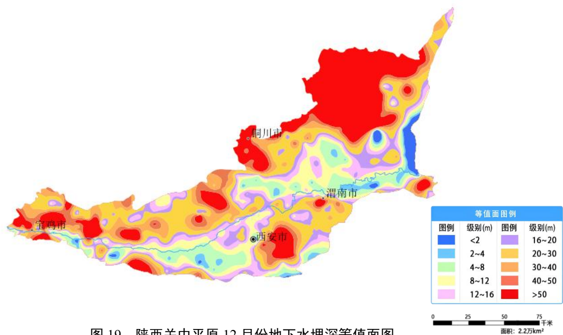
图 19 陕西关中平原 12 月份地下水埋深等值面图
