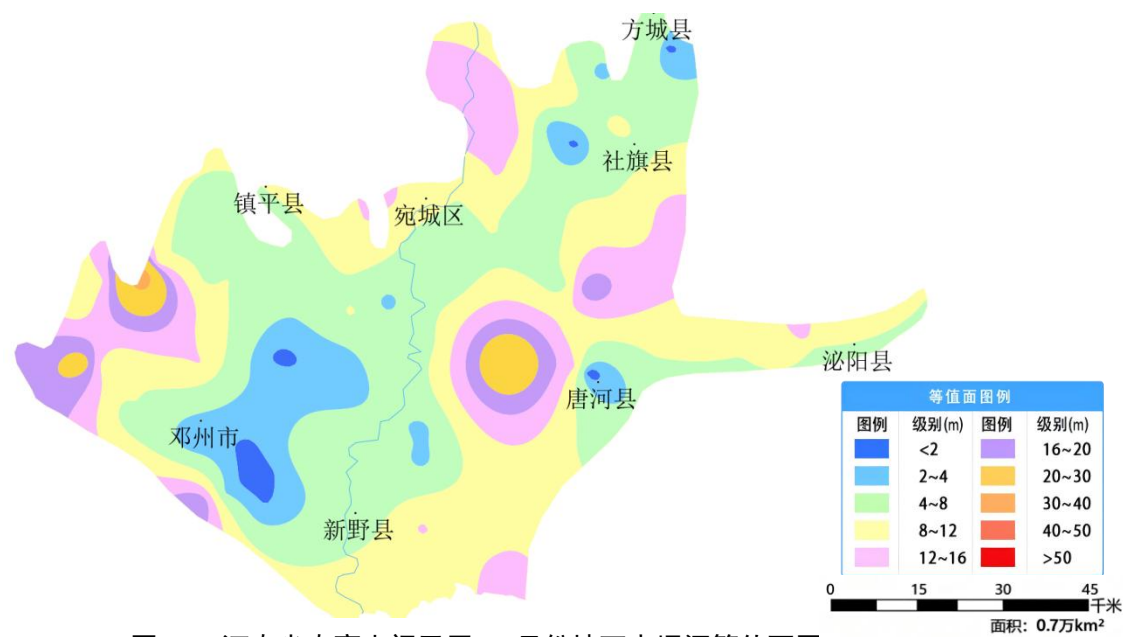
图 31 河南省南襄山间平原 12 月份地下水埋深等值面图
