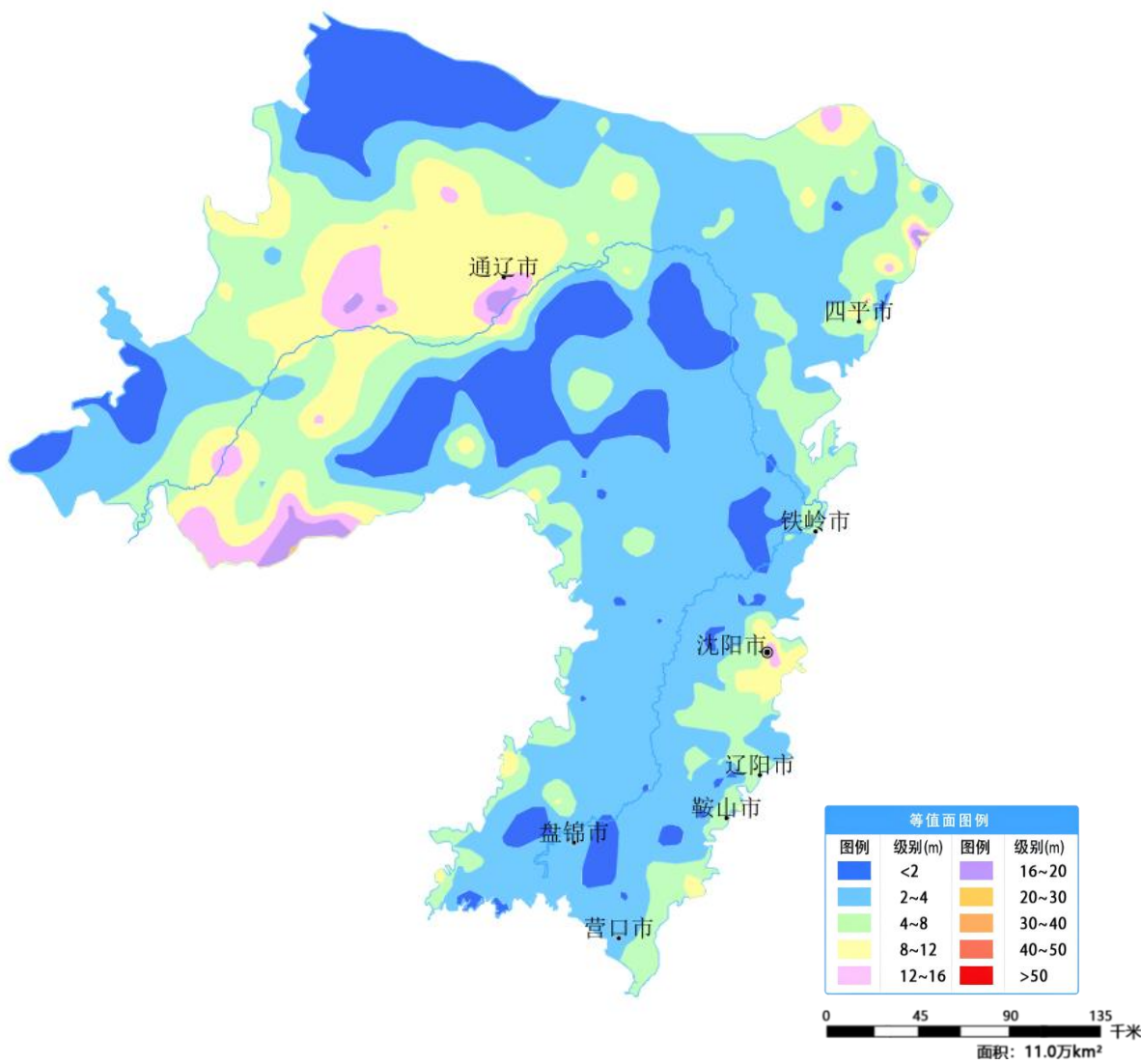
图 7 辽河平原 12 月份地下水埋深等值面图
