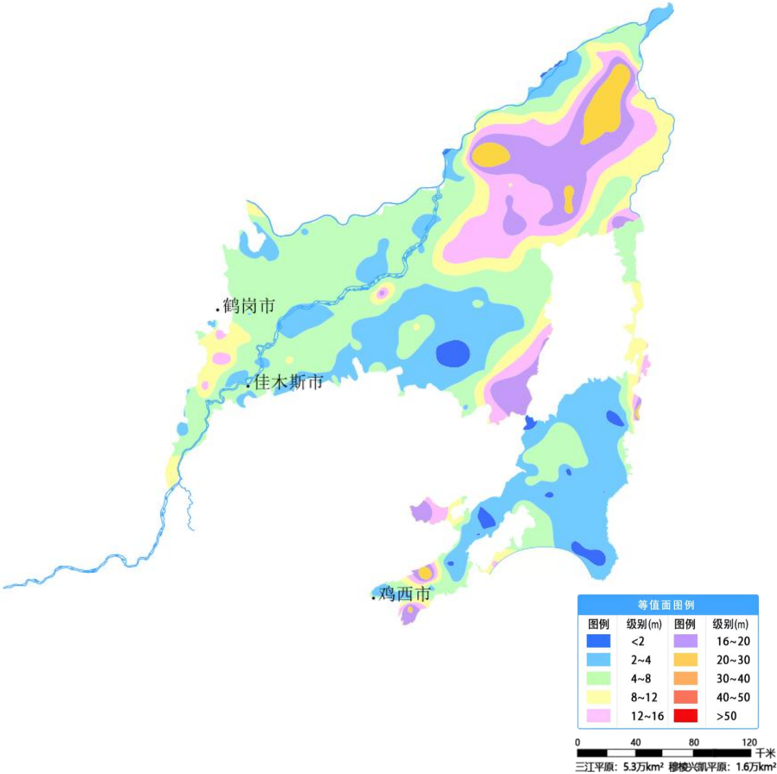
图 1 三江平原和穆棱兴凯平原 12 月份地下水埋深等值面图
