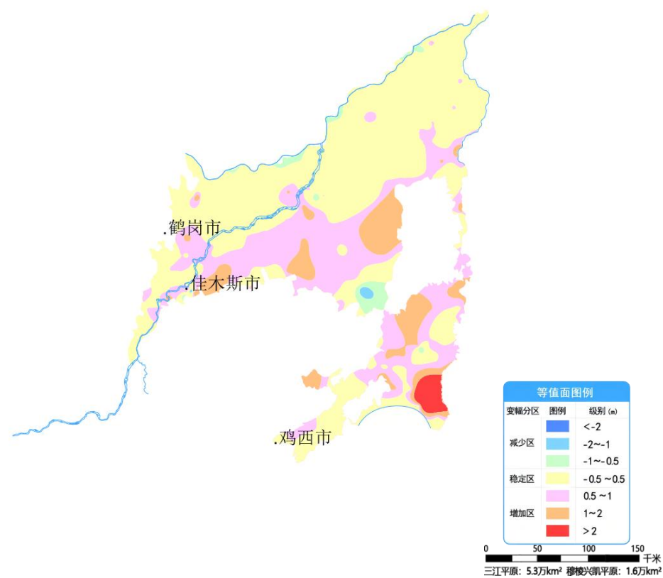
图 3 三江平原和穆棱兴凯平原 11 月份与去年同期相比地下水埋深变幅图
