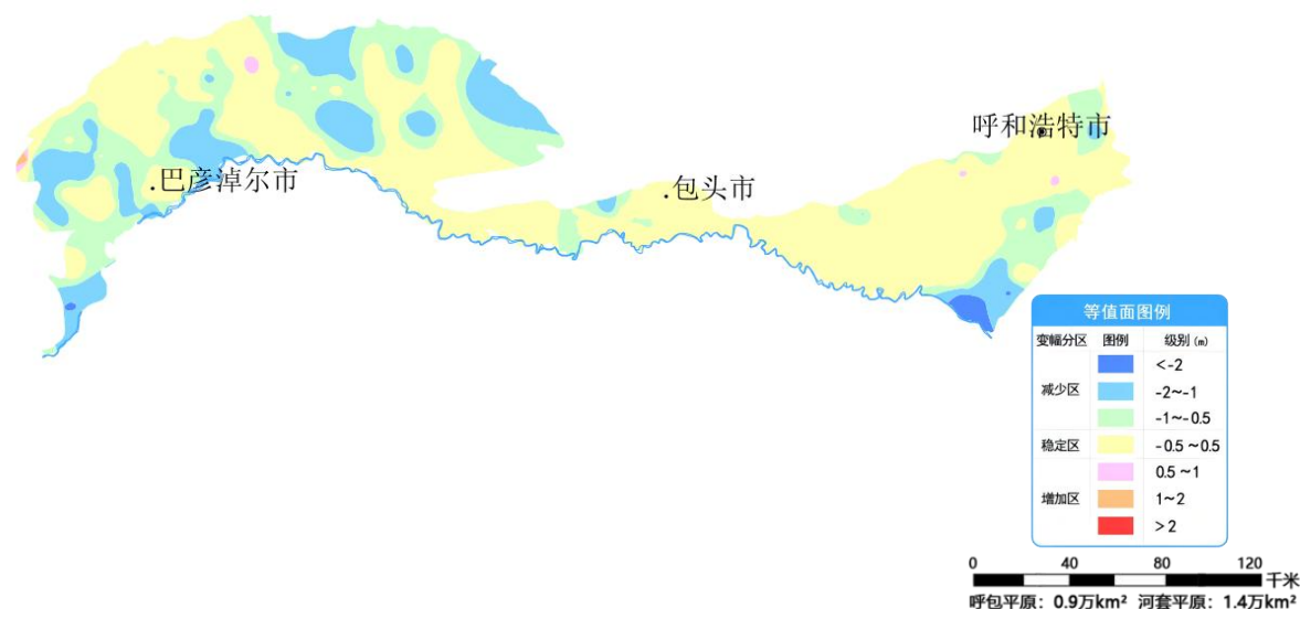
图 17 内蒙古呼包平原及河套平原 11 月份与上月相比地下水埋深变幅图
