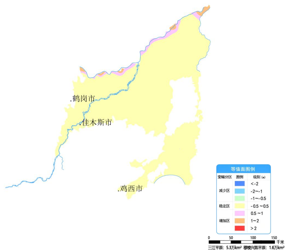
图 2 三江平原和穆棱兴凯平原 11 月份与上月相比地下水埋深变幅图
