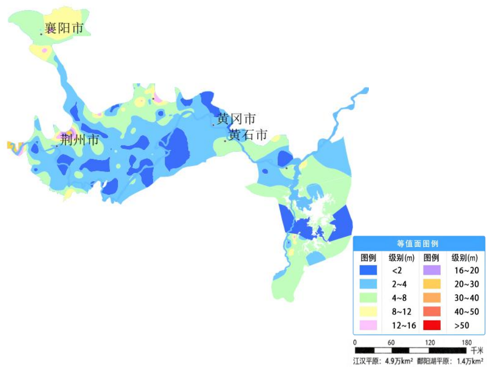
图 29 江汉平原和鄱阳湖平原 11 月份地下水埋深等值面图
