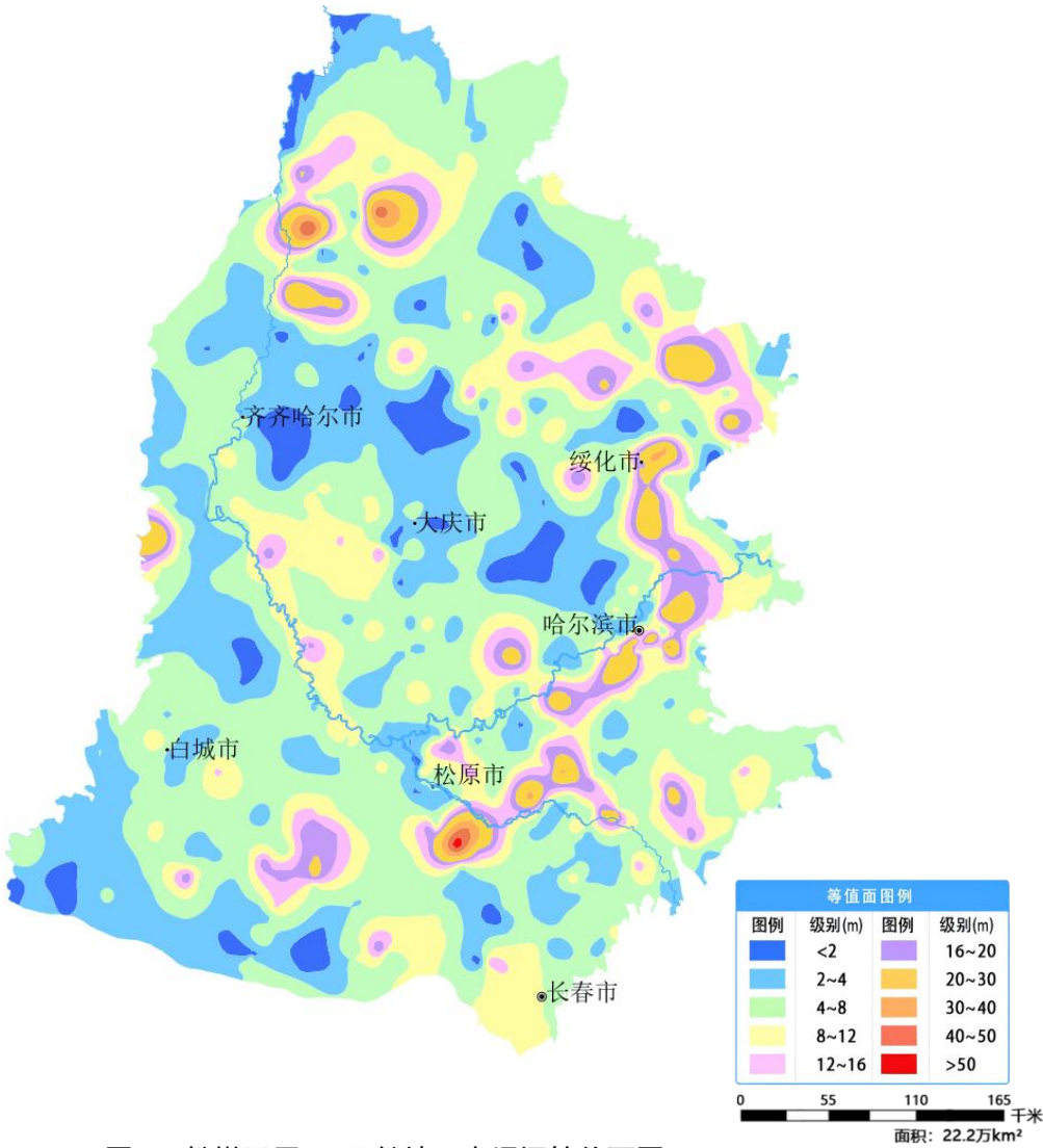
图 4 松嫩平原 11 月份地下水埋深等值面图
