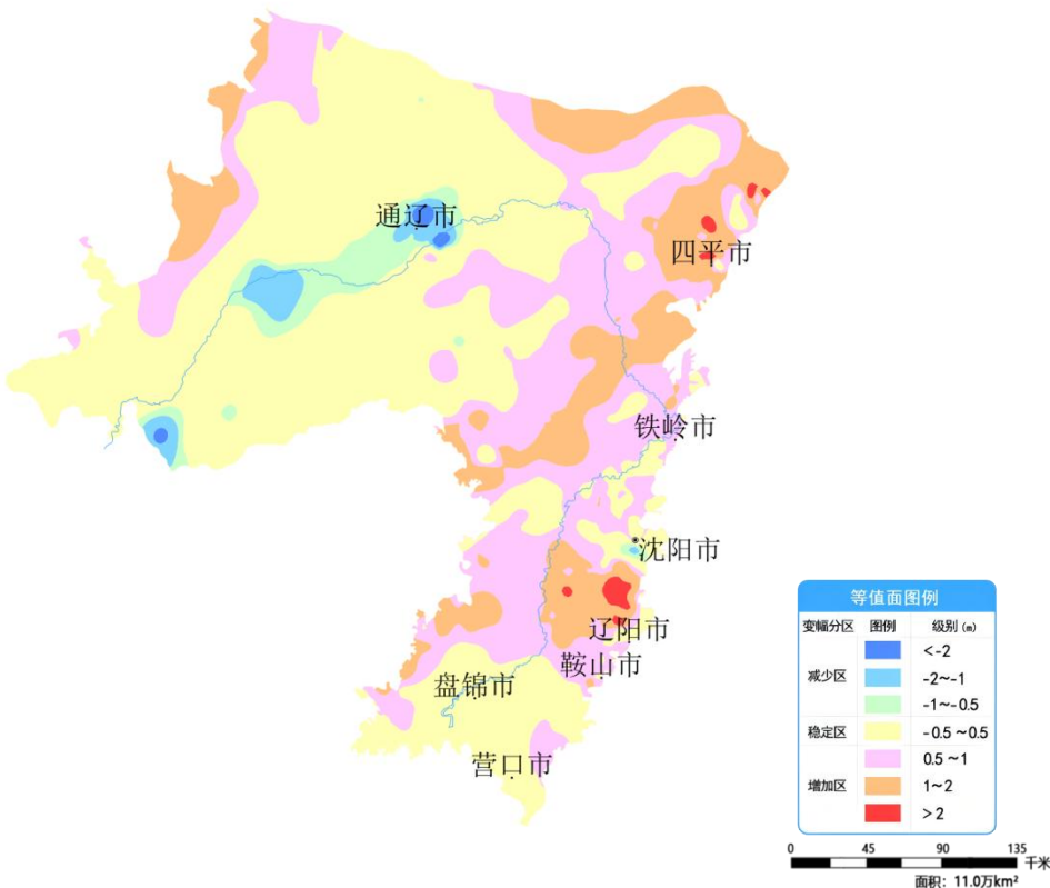
图 9 辽河平原 11 月份与去年同期相比地下水埋深变幅图
