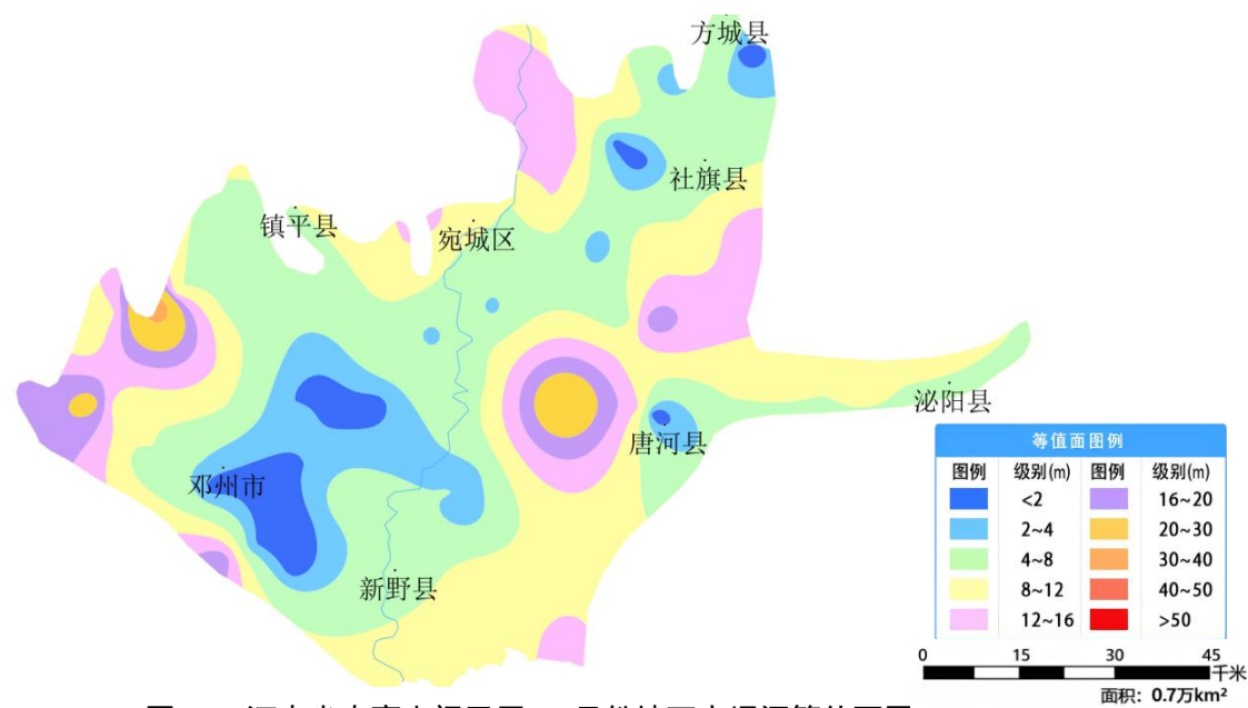
图 31 河南省南襄山间平原 11 月份地下水埋深等值面图
