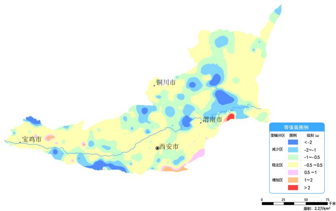
图 20 陕西关中平原 11 月份与上月相比地下水埋深变幅图
