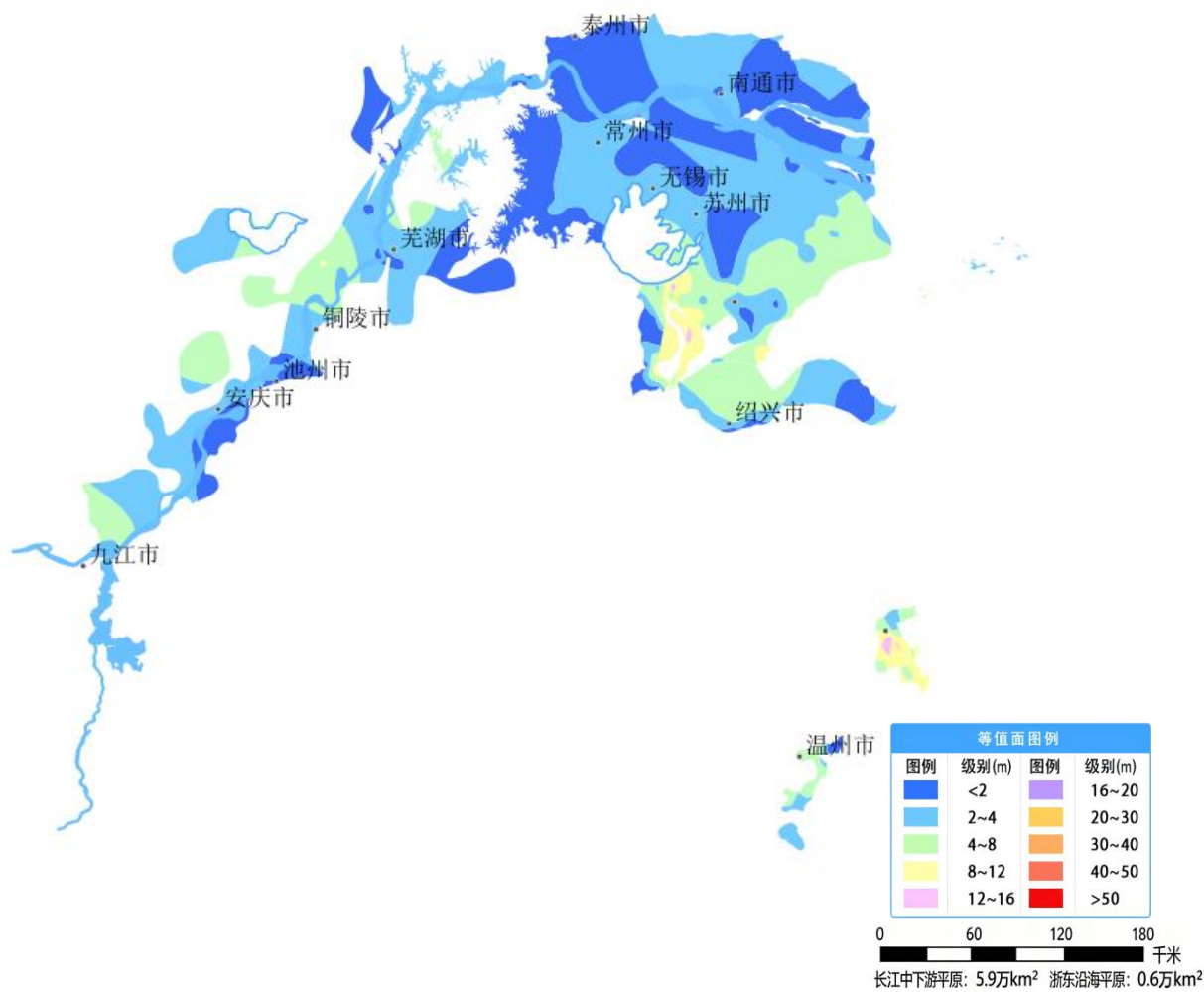
图 30 长江三角洲平原和浙东沿海平原 11 月份地下水埋深等值面图
