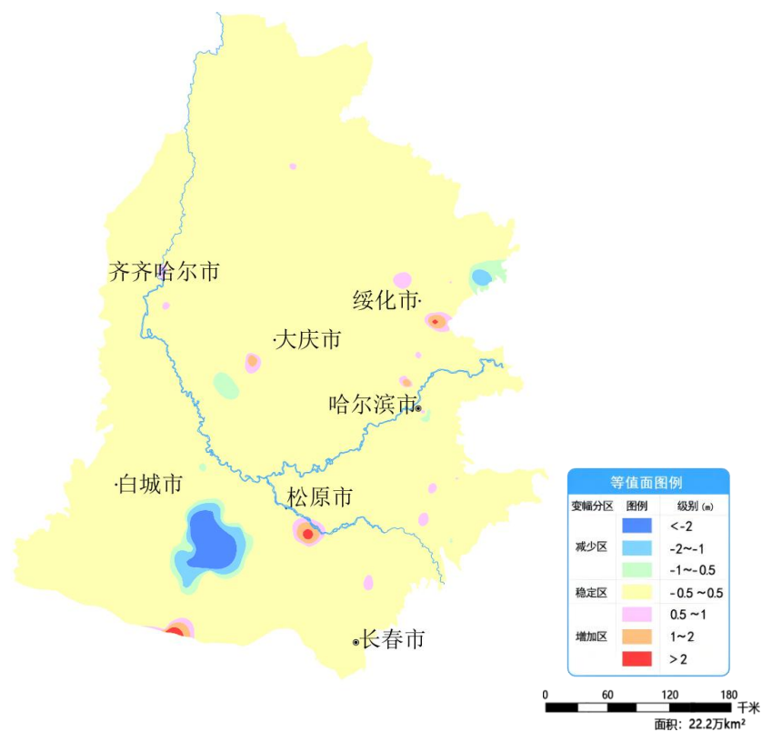
图 5 松嫩平原 11 月份与上月相比地下水埋深变幅图
