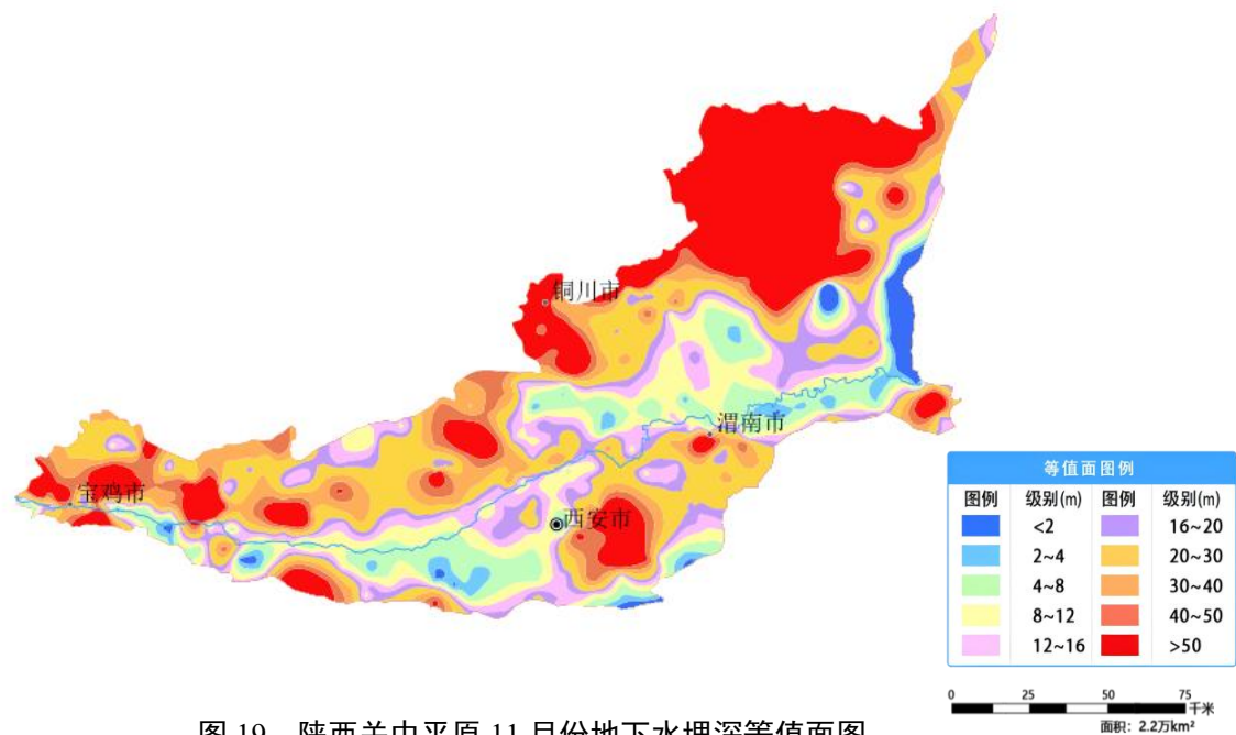
图 19 陕西关中平原 11 月份地下水埋深等值面图
