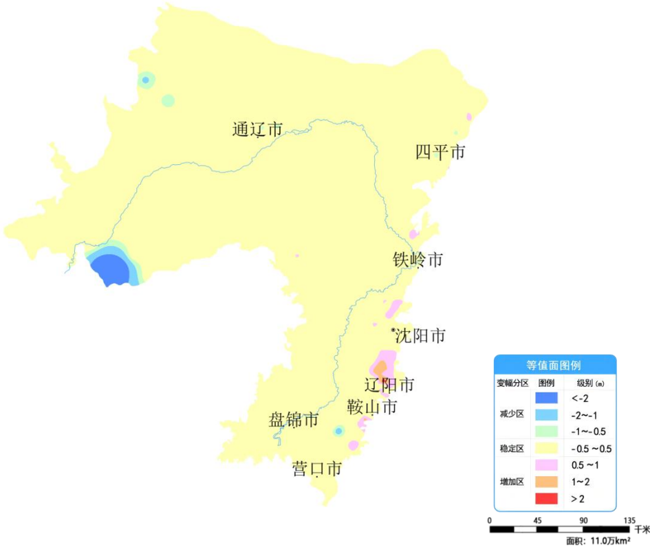
图 8 辽河平原 11 月份与上月相比地下水埋深变幅图
