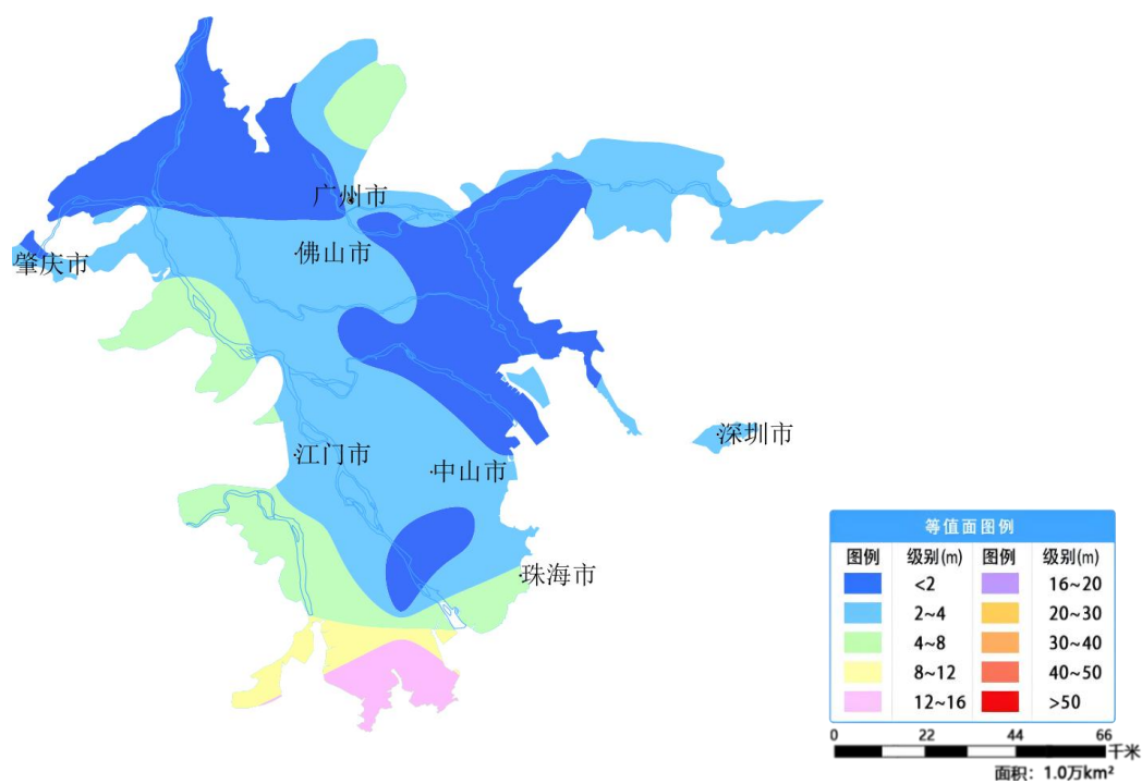
图 33 广东珠江三角洲平原 11 月份地下水埋深等值面图
