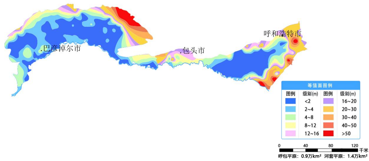
图 16 内蒙古呼包平原及河套平原 11 月份地下水埋深等值面图
