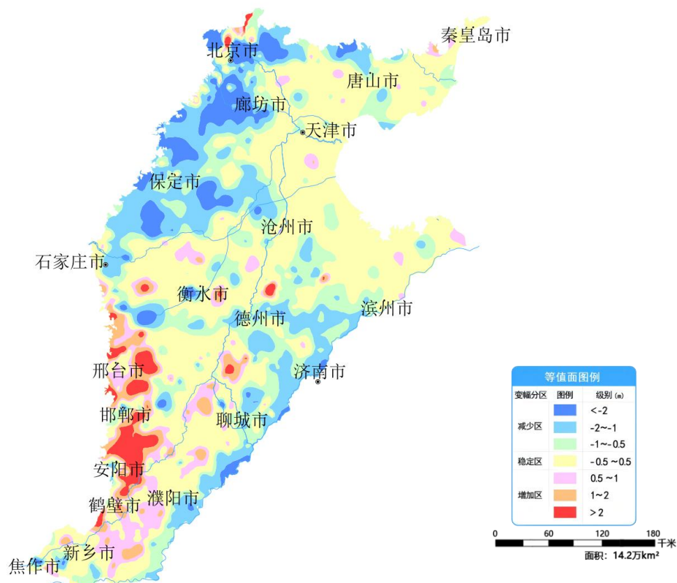
图 12 海河平原 11 月份与去年同期相比地下水埋深变幅图
