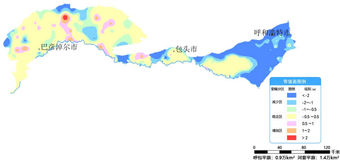
图 18 内蒙古呼包平原及河套平原 11 月份与去年同期相比地下水埋深变幅图
