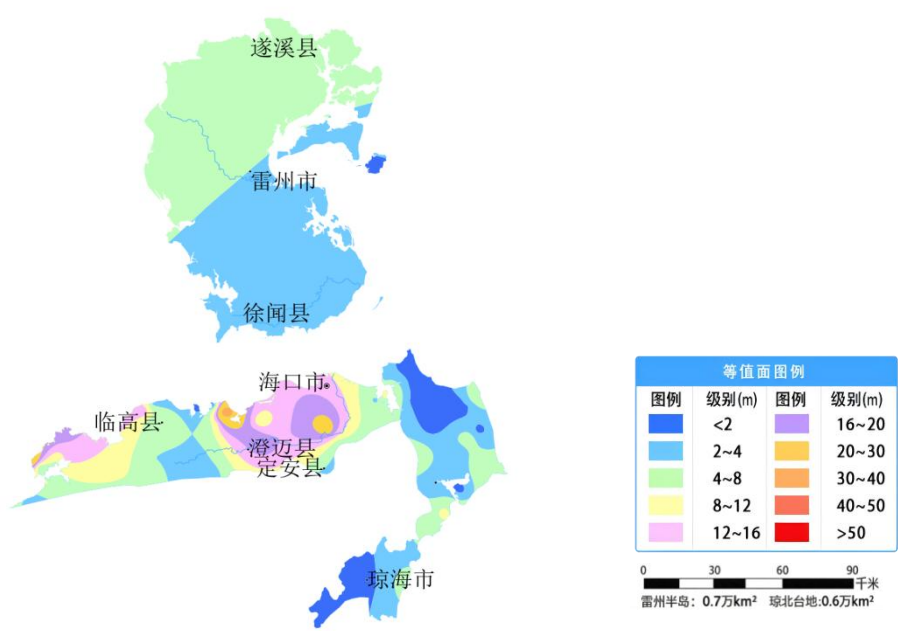
图 34 雷州半岛平原和琼北台地平原 11 月份地下水埋深等值面图
