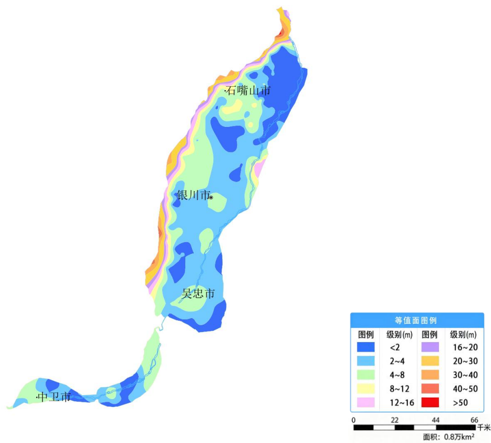
图 25 宁夏银川卫宁平原 11 月份地下水埋深等值面图
