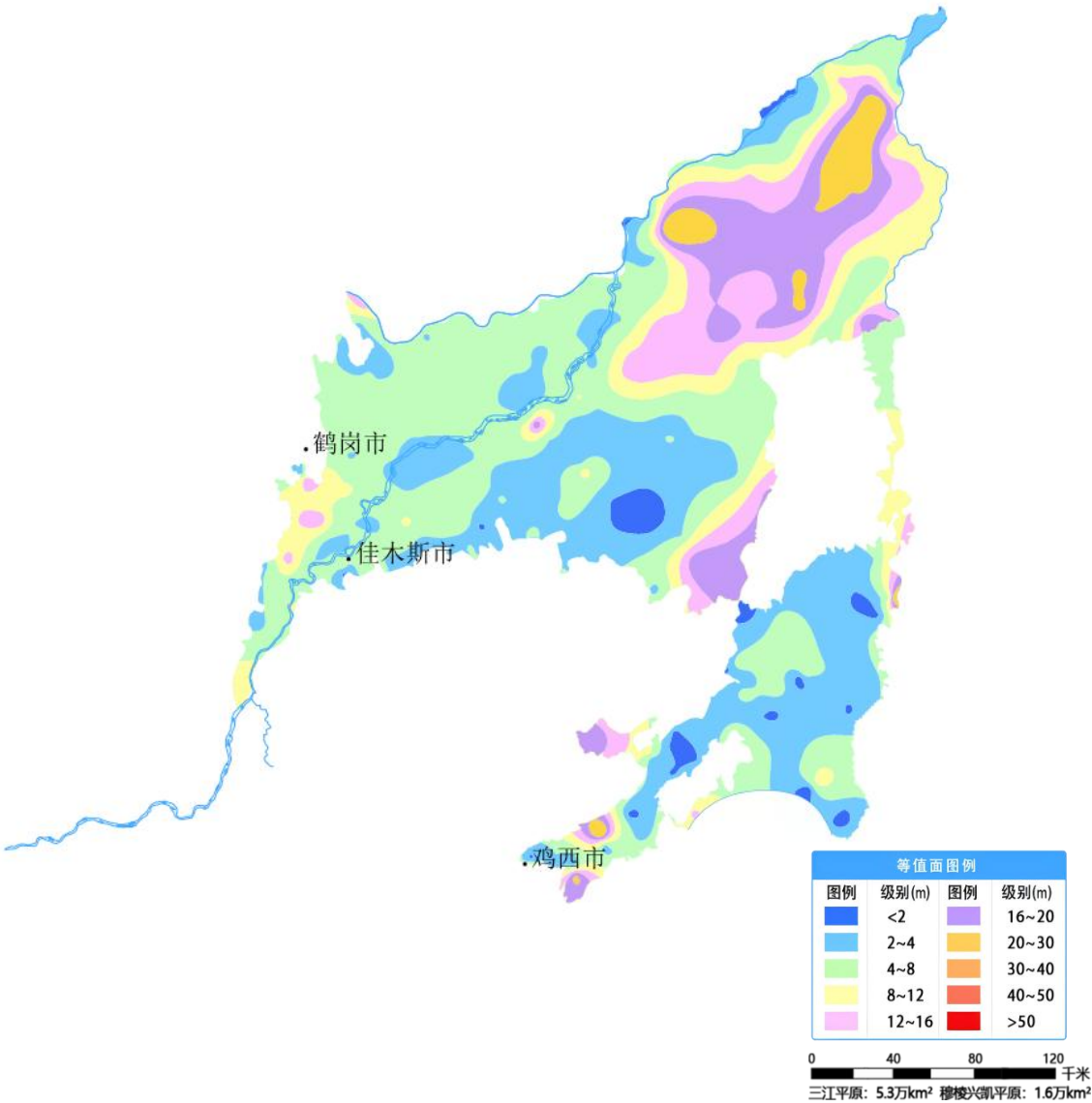
图 1 三江平原和穆棱兴凯平原 11 月份地下水埋深等值面图
