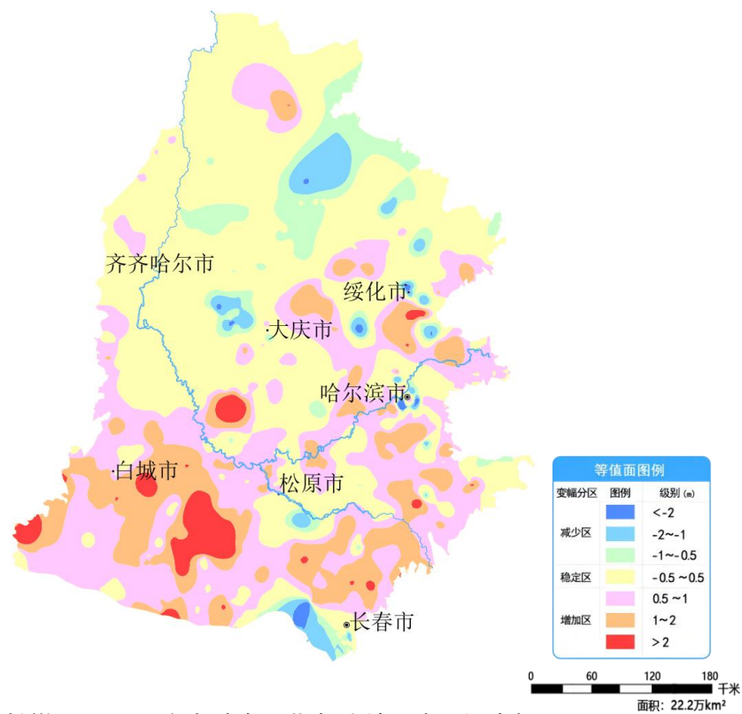
图 6 松嫩平原 11 月份与去年同期相比地下水埋深变幅图
