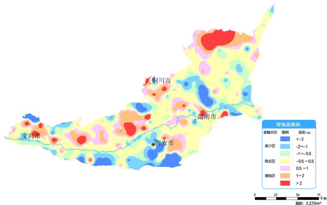
图 21 陕西关中平原 11 月份与去年同期相比地下水埋深变幅图
