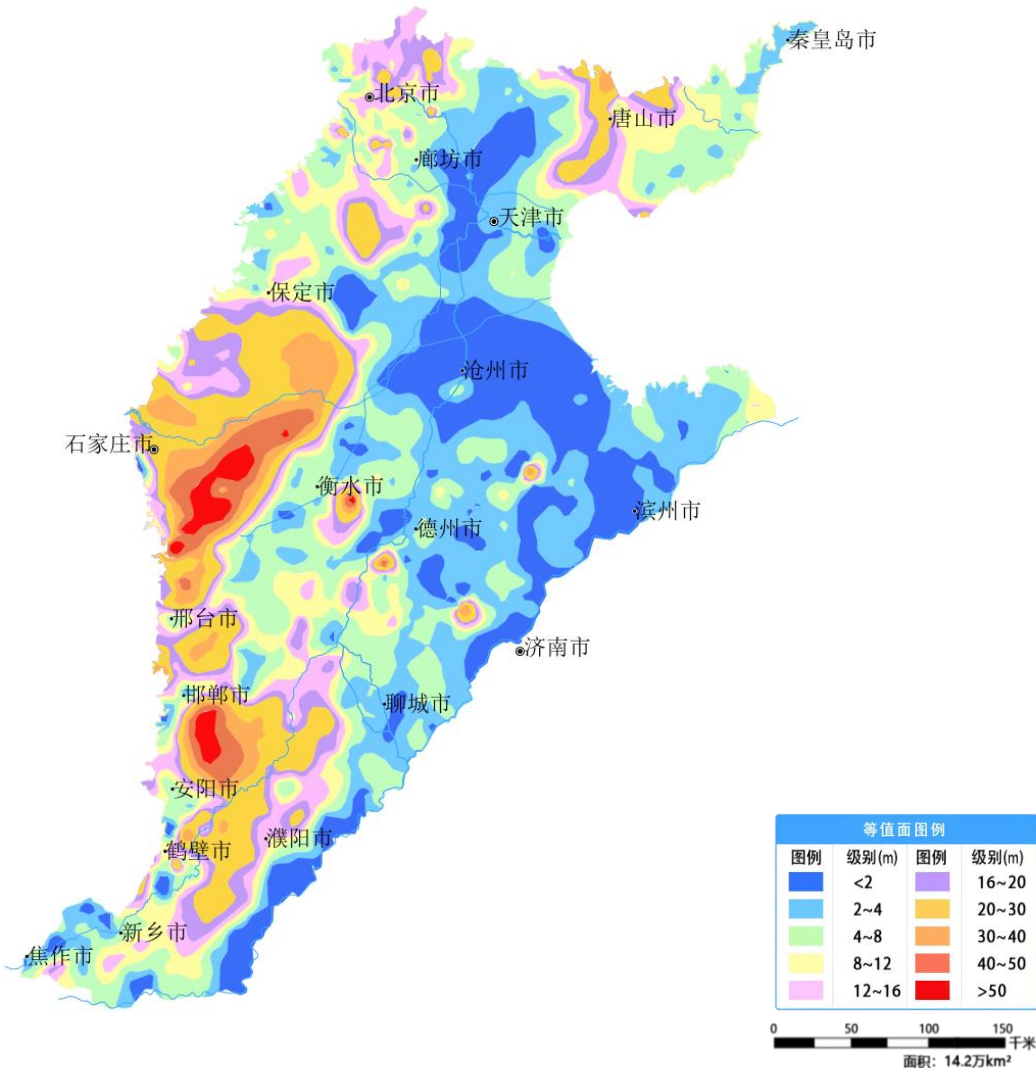
图 10 海河平原 11 月份地下水埋深等值面图
