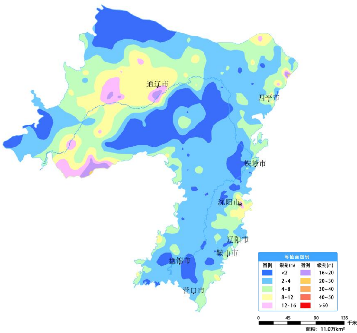
图 7 辽河平原 11 月份地下水埋深等值面图
