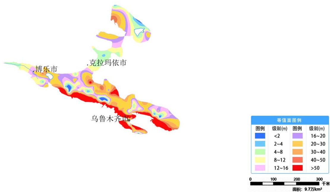
图 28 新疆准噶尔盆地监控区 11 月份地下水埋深等值面图
