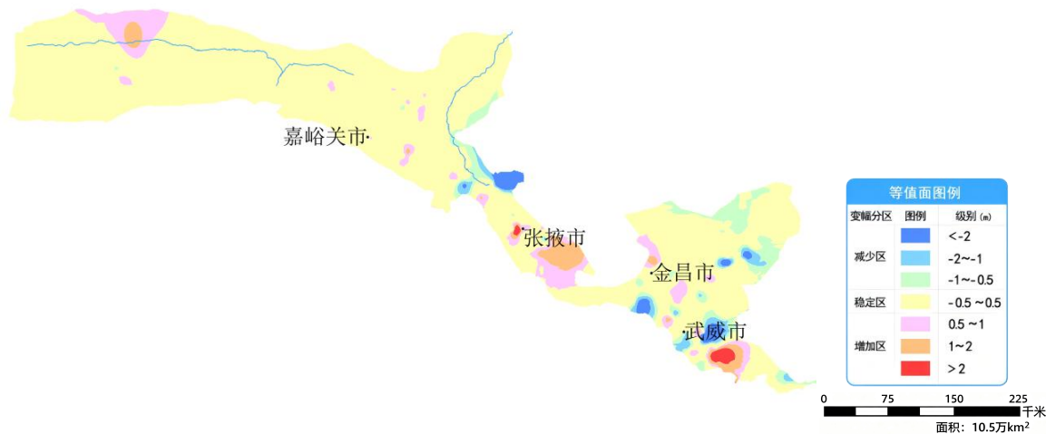
图 24 甘肃河西走廊平原 11 月份与去年同期相比地下水埋深变幅图
