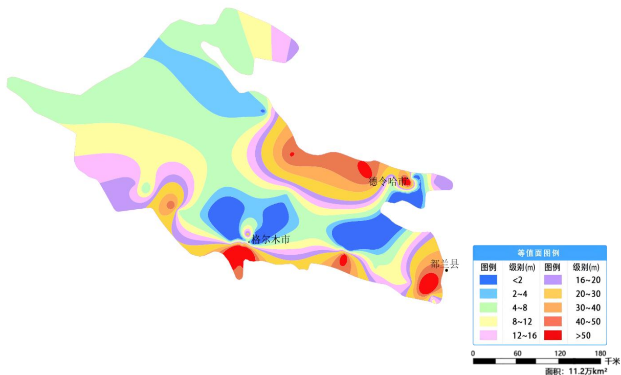
图 26 青海柴达木盆地 11 月份地下水埋深等值面图
