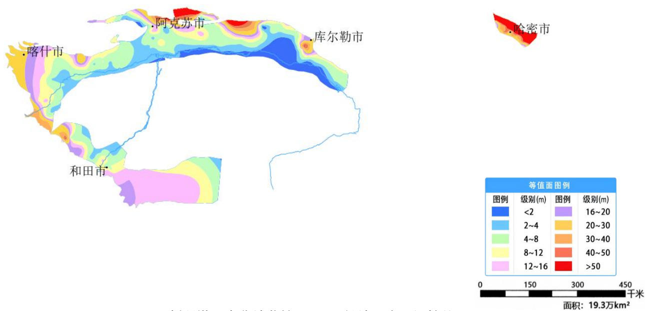
图 27 新疆塔里木盆地监控区 11 月份地下水埋深等值面图
