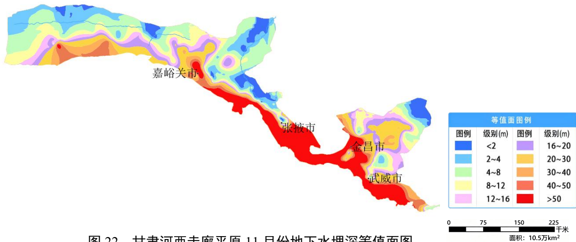
图 22 甘肃河西走廊平原 11 月份地下水埋深等值面图
