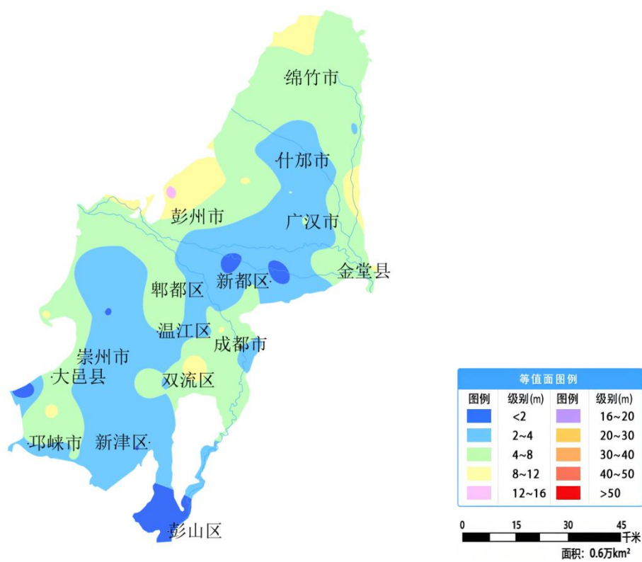
图 32 成都平原 11 月份地下水埋深等值面图
