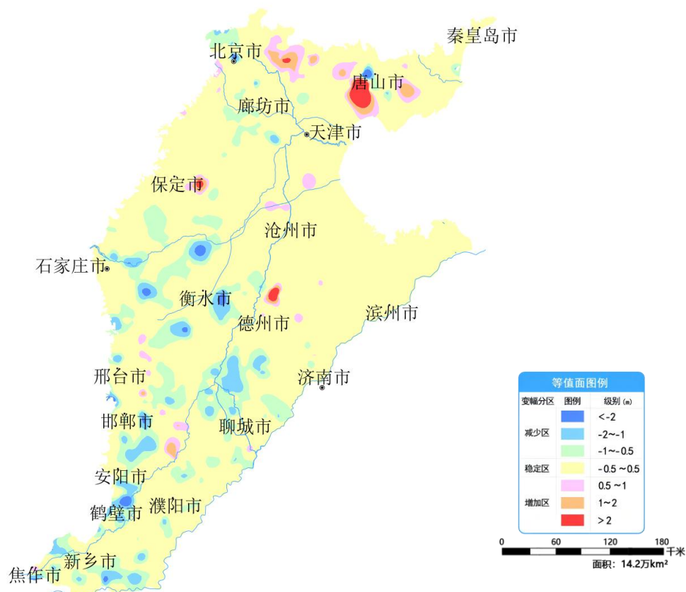
图 11 海河平原 11 月份与上月相比地下水埋深变幅图
