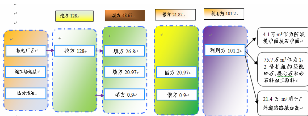
图 3.2-1 土石方平衡图
