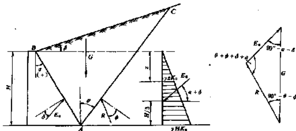
图 3.2-1 库仑主动土压力计算图
